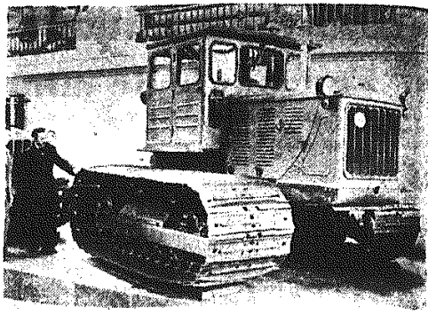
Nowe maszyny dla rolnictwa. Na zdjęciu: nowy traktor gatunkowy Dniepr (na górnym podwoziu). Szerokość gąsienic - 1000 mm, ciśnienie na grunt - 0,25 kg na 1 cm 2 , liczba biegów - 4 (w tym 2 wsteczne).
